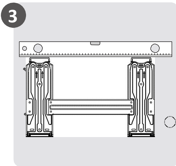
Anbringen der Montageplatte (Seite 12)
