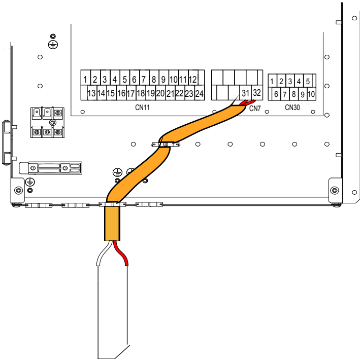
ABTAUANFORDERUNGSSIGNAL
